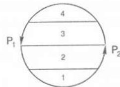
Figur 3b: die gleichzeitige vertikale Reflexionsstufung
