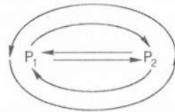
Figur 2d: vereinfachte Schematisierung der doppelt-gegenläufigen Reflexion
